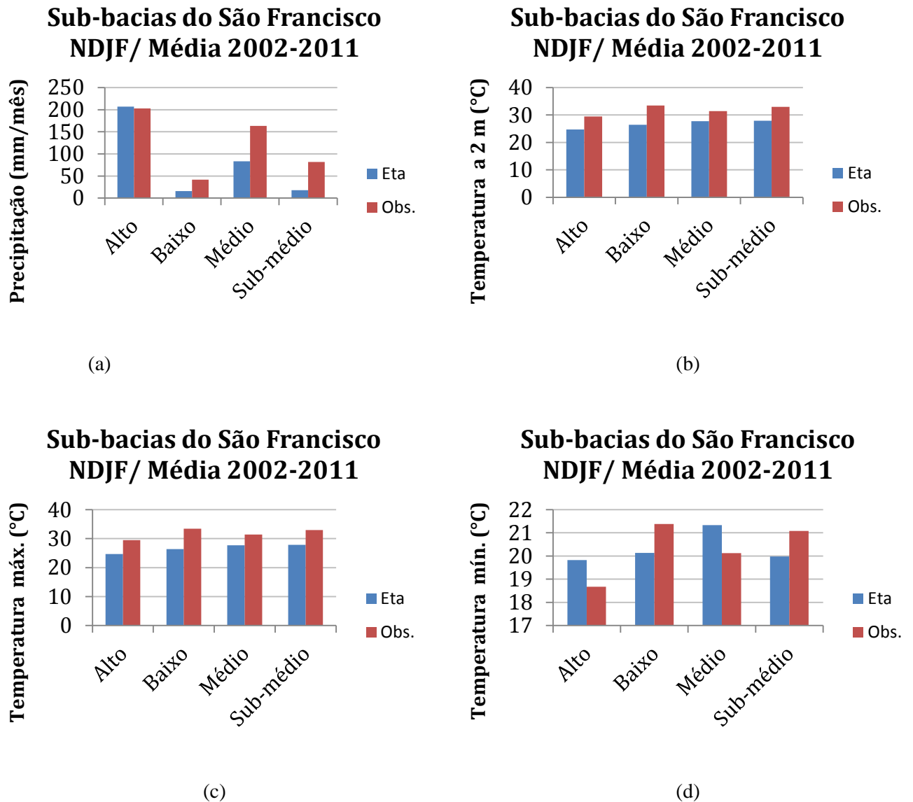
Figura 5.5 – Gráficos da média do modelo Eta e do Observado dos quatro meses
