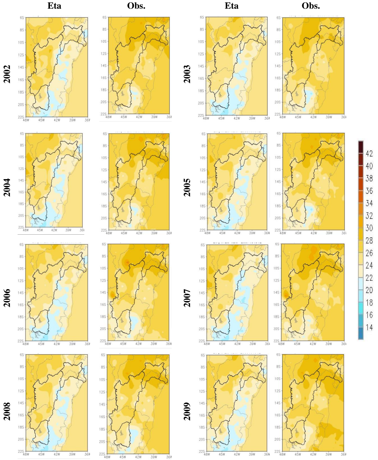
Figura 5.4 – Temperatura a 2 metros média sazonal (°C) previsão do Modelo Regional do Eta, média no período 2002-2012
