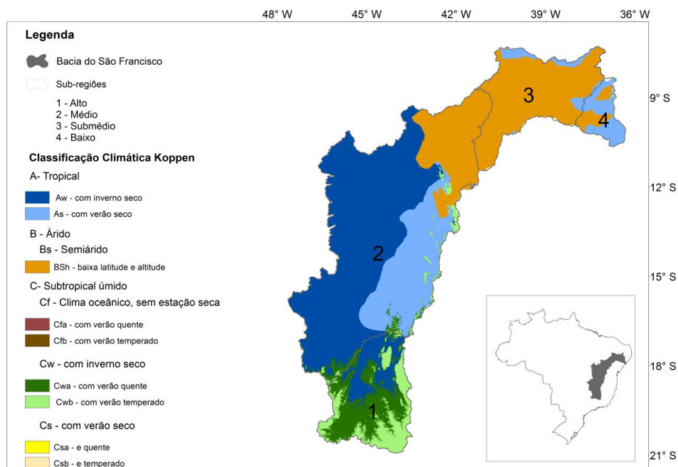
Figura 2.1 – Região Hidrográfica do São Francisco e classificação climática de Koppen.
